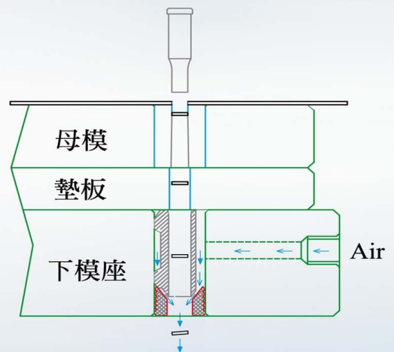
吸料銷運作示意圖 (單孔時, 使用)
