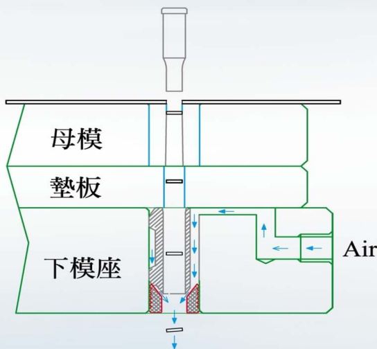
吸料銷運作示意圖 (多孔時, 使用)
